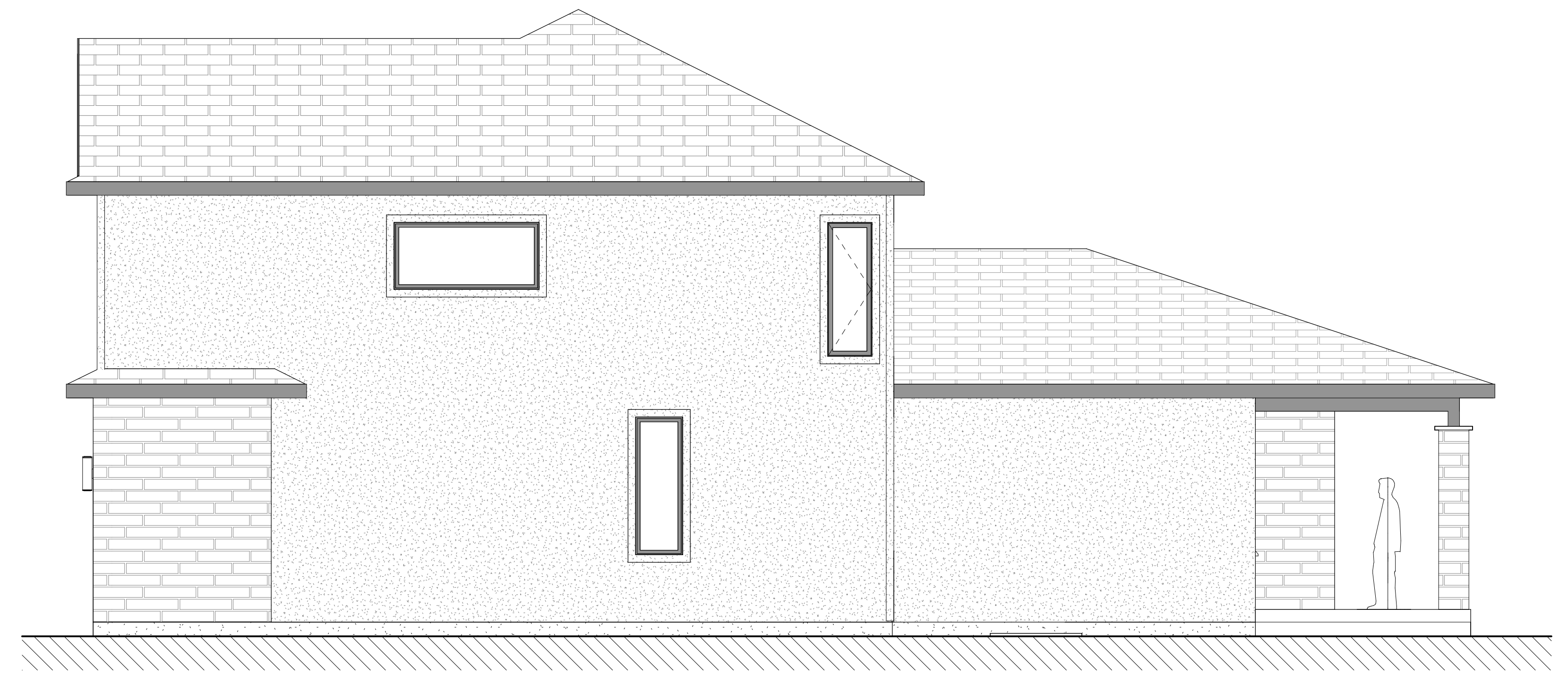
RIGHT ELEVATION
