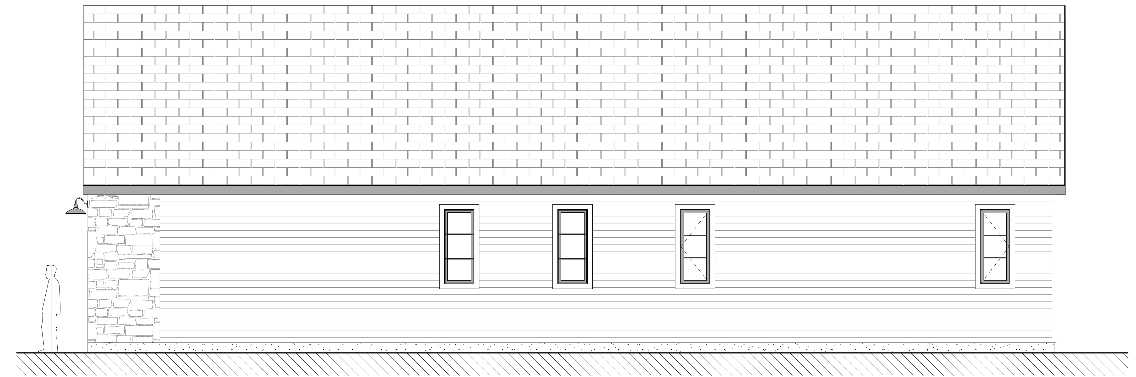
RIGHT ELEVATION
